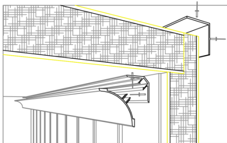
ขยาย การยึดแผ่นฝ้า+ผนัง (ด้านริม)
