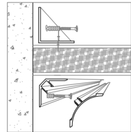
ขยาย การยึดฝ้า+ผนังคอนกรีต DETAIL FOR CONCRETE WALL & CEILING
