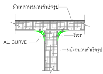
ขยาย การยึดแผ่นฝ้า+ผนัง (ช่วงกลาง)
