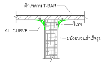
ขยาย การยึดผนัง + แผ่นฝ้า (T-BAR)
