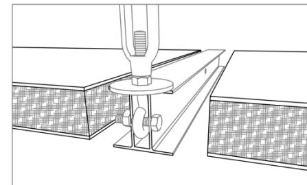
จุดหนีว "H" รอยต่อแผ่นเพดาน
