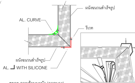
ขยาย การเข้ามุมผนัง (จากข้าง) DETAIL FOR WALL & WALL AT CORNER
